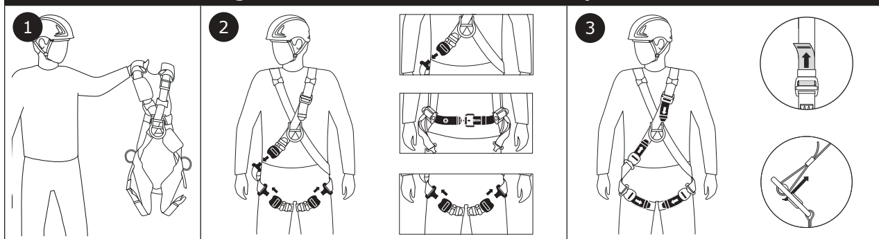
Figure 6B - Enfillement du harnais de style croisé
