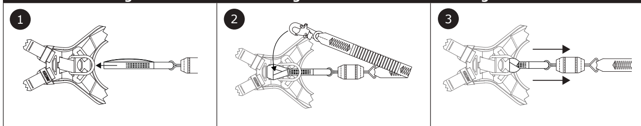
Figure 13 - Fixation des longes avec des boucles d'étranglement
