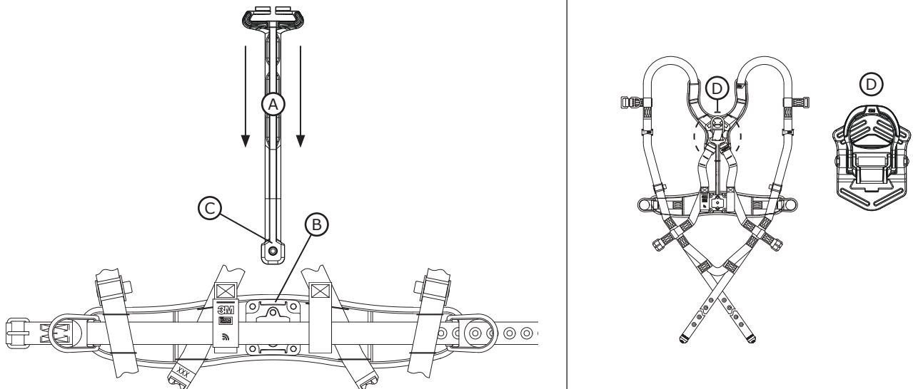
Figure 11 - Fixation du système de répartition du poids
