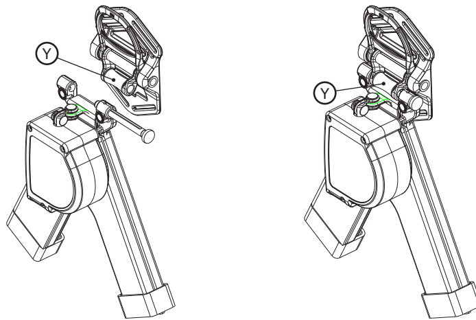
Figure 10D - Adaptateur à dispositif autorétractable
