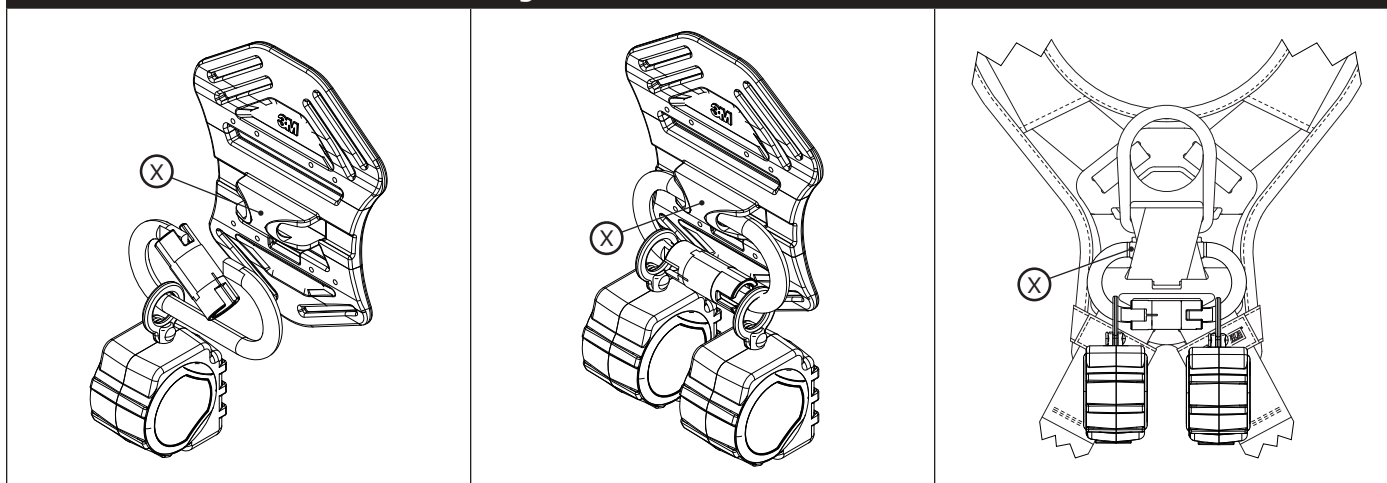
Figure 10C - Boucle d'interface
